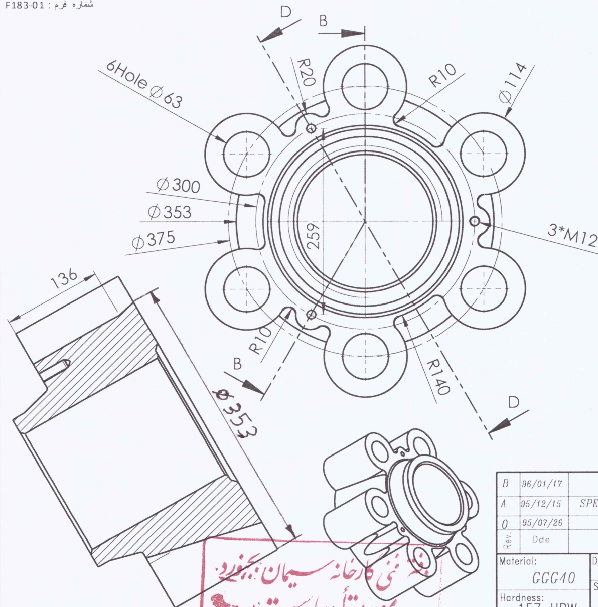
SECTION D-D SCALE 1 : 5
