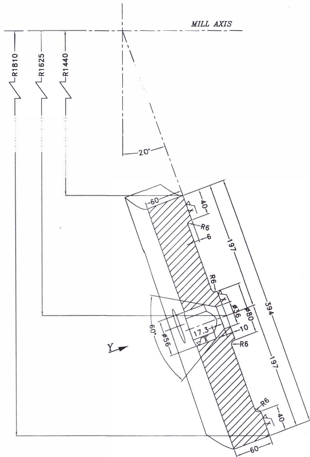
SEC. A-A
