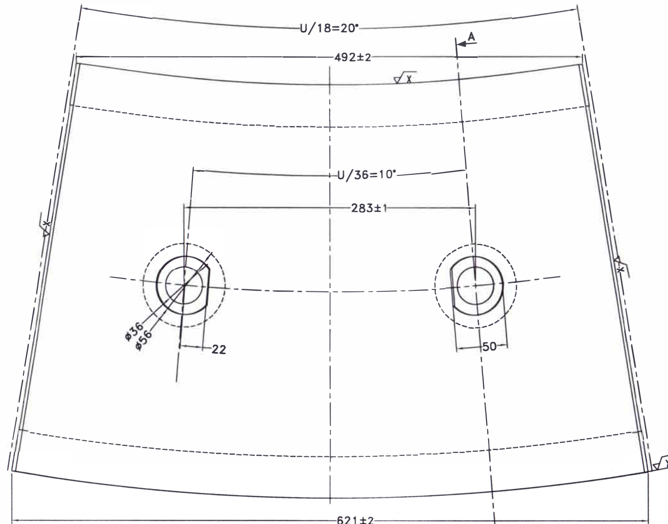
VIEW Y
