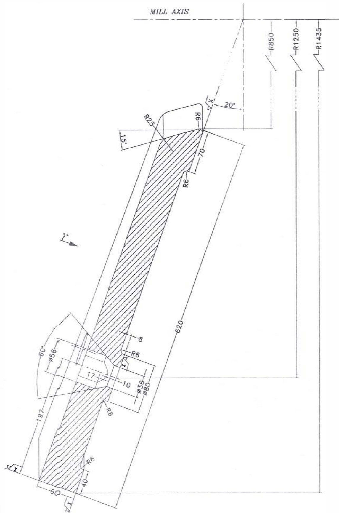
SEC. A-A
