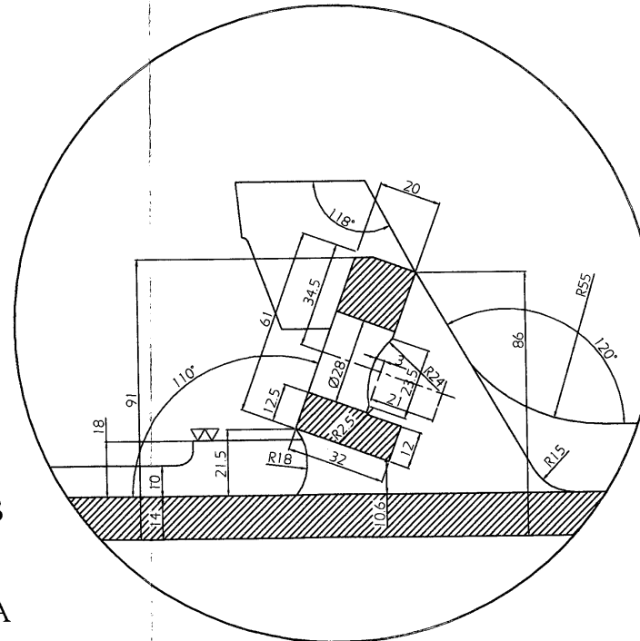
Detail: Z
