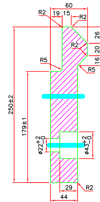
SECTION A-A
