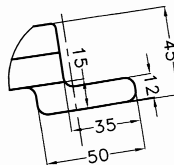
View Y Scale 1:2
