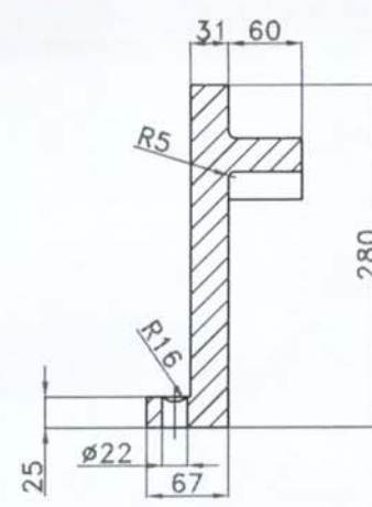
Sec. A-A
