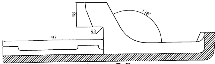
Section:B-B
