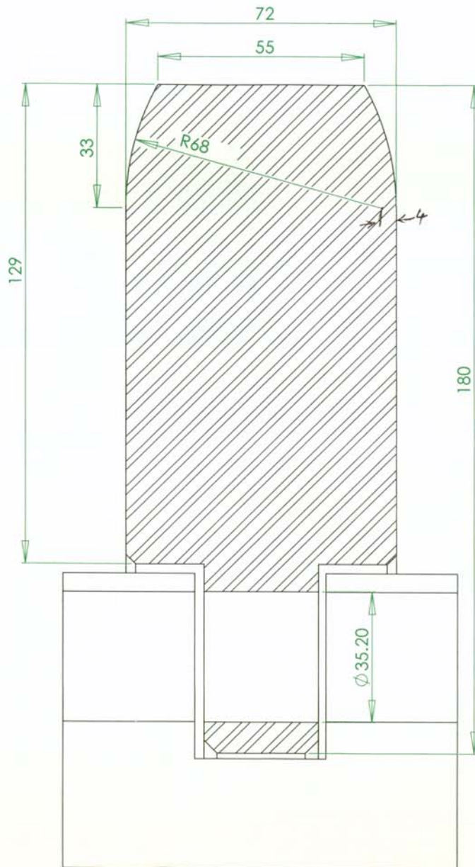
SECTION A-A SCALE 1:1
